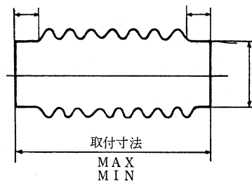
丸型フランジ無し
